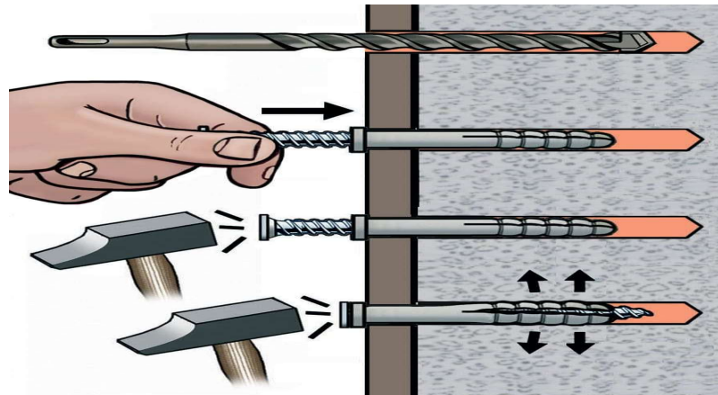
CHEVILLE DE FRAPPE
